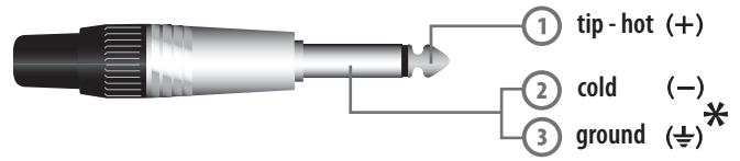
INPUT Jack (unbalanced) INPUT (ingresso) Jack (sbilanciato)
